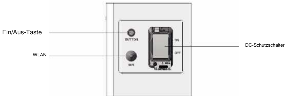
Abbildung 2-2-2 Linke Seite des Steuerungsmoduls
