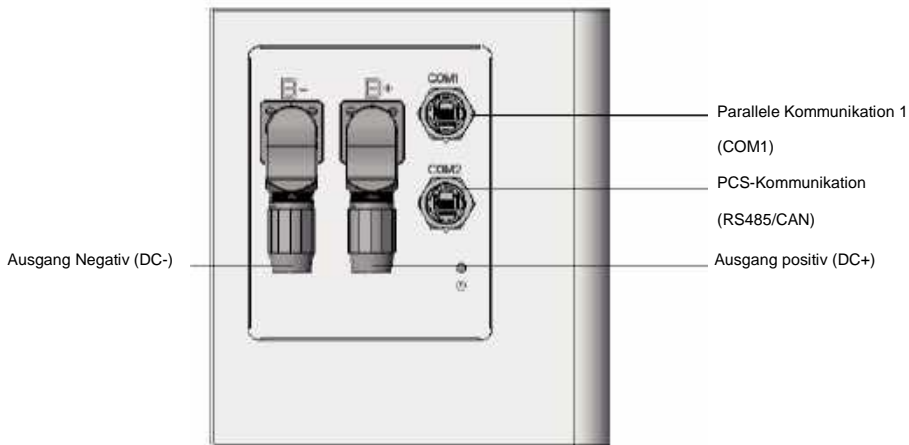
Abbildung 2-2-3 Steuermodul
