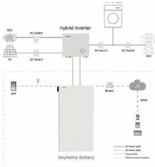
Abbildung 2-1-2 Systemtopologie
